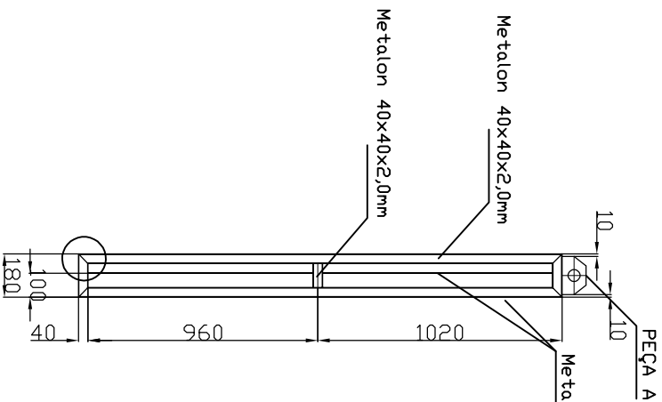
VISTA LATERAL
