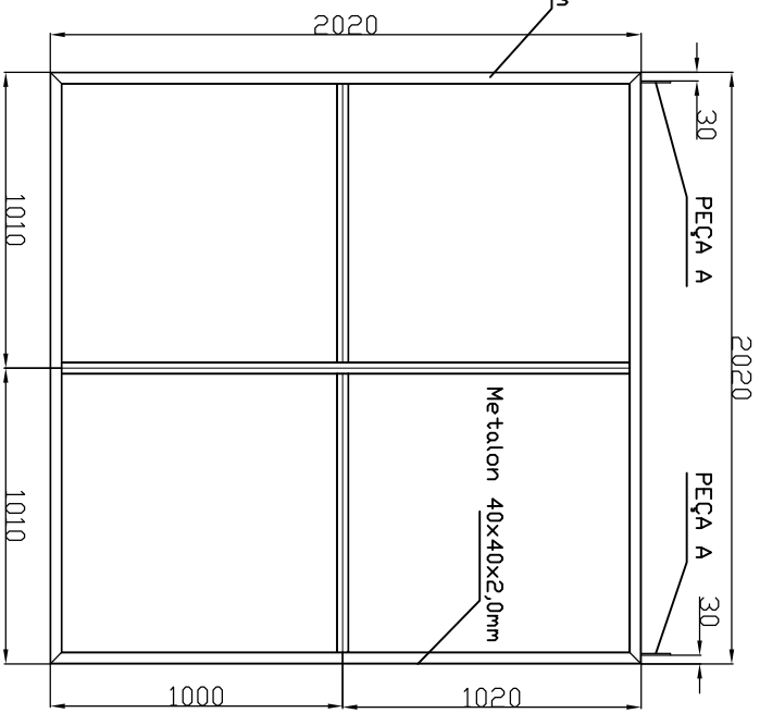
VISTA DO FUNDO
